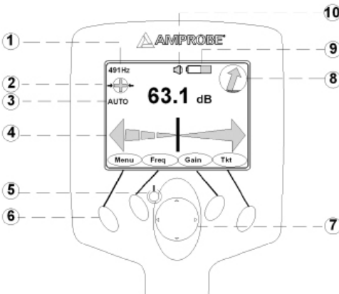
R-5000 Bedienungsfläche
