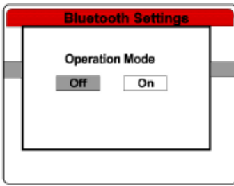
T-5000-Bluetooth-Betriebsmodus
